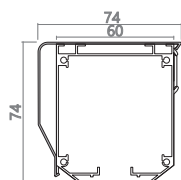
Przekrój rynny
