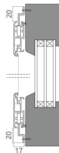
z prowadnicami typu A
