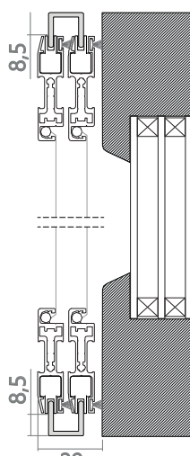
z prowadnicami typu B
